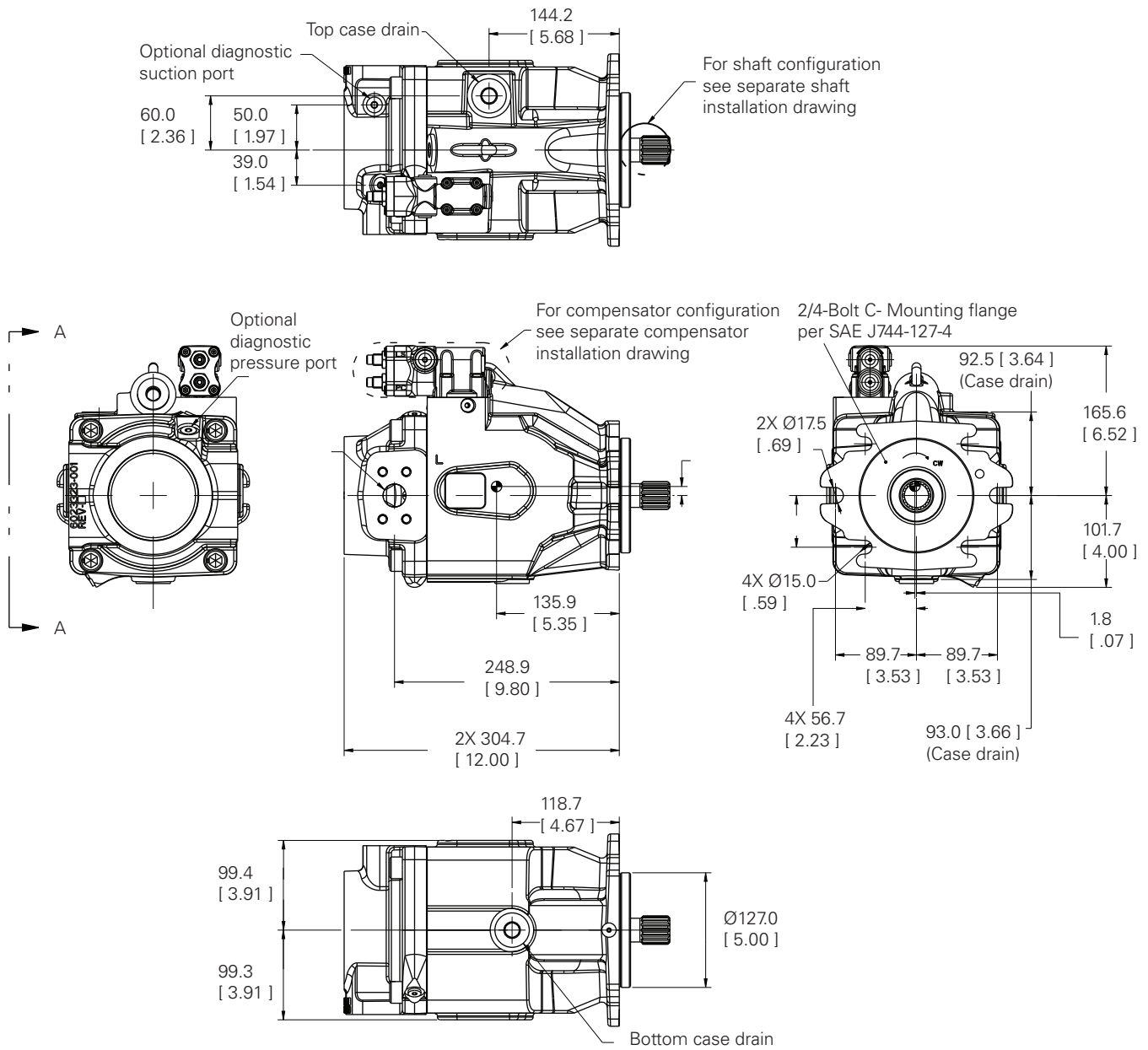
View A-A
