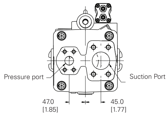
LH Rotation
