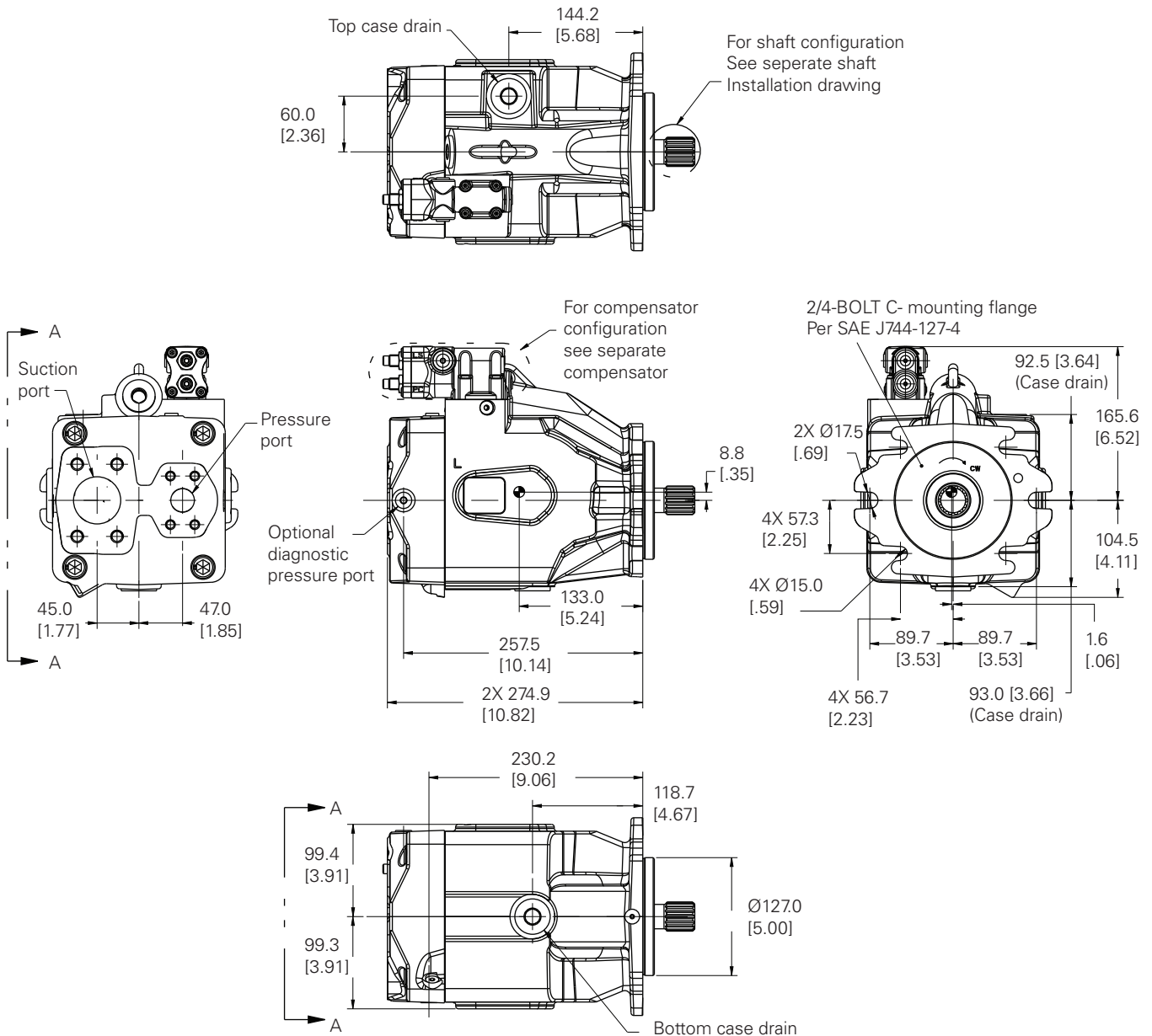
View A-A
