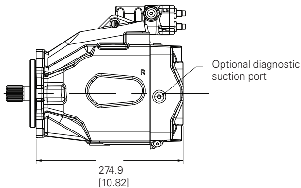
View A-A
